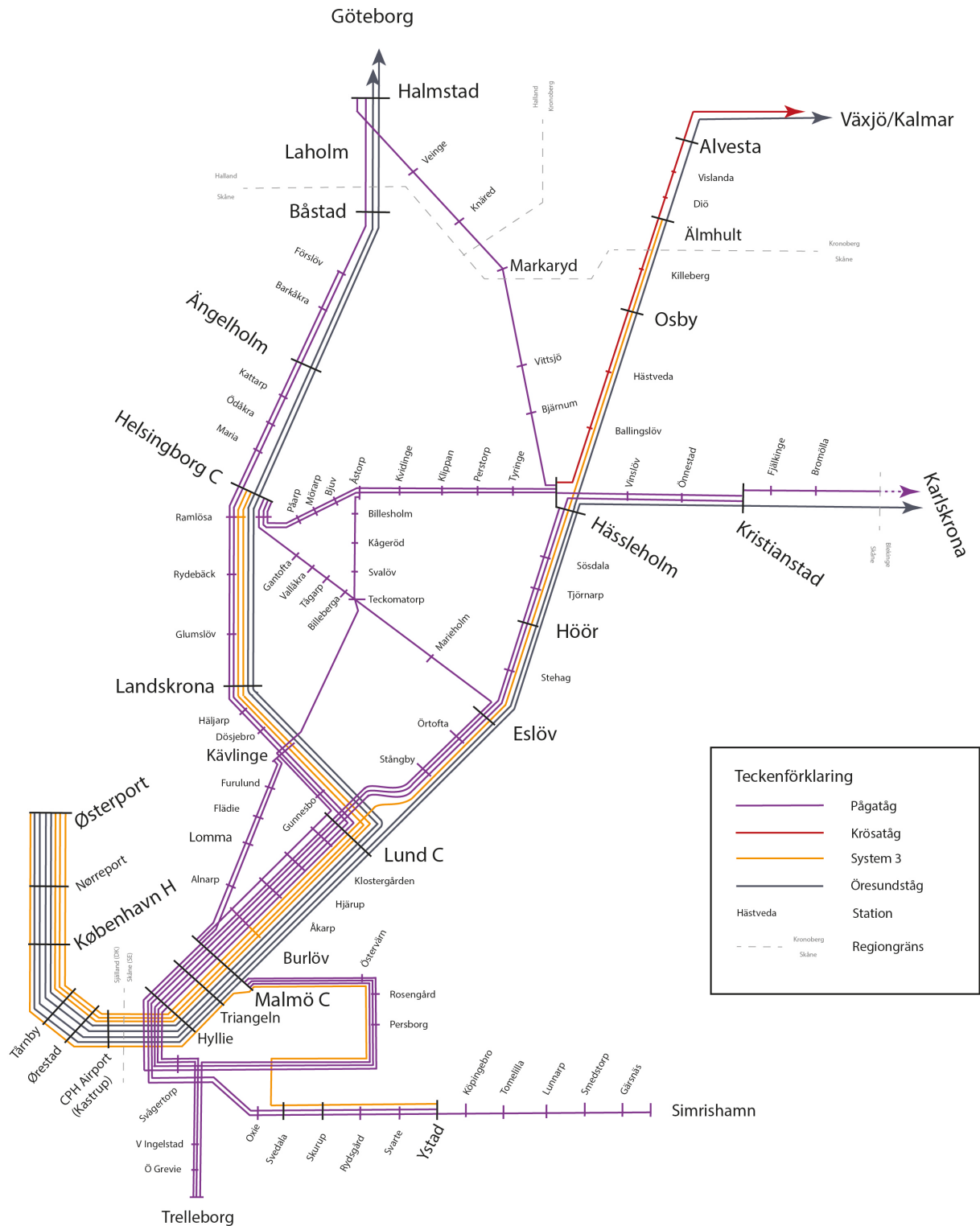
Figur 17: Schematisk bild över behov av tågtrafik för att nå målen år 2030. Exklusive fjärrtåg och godståg. En linje innebär ett tåg per timme i vardera riktningen i högtrafik.
