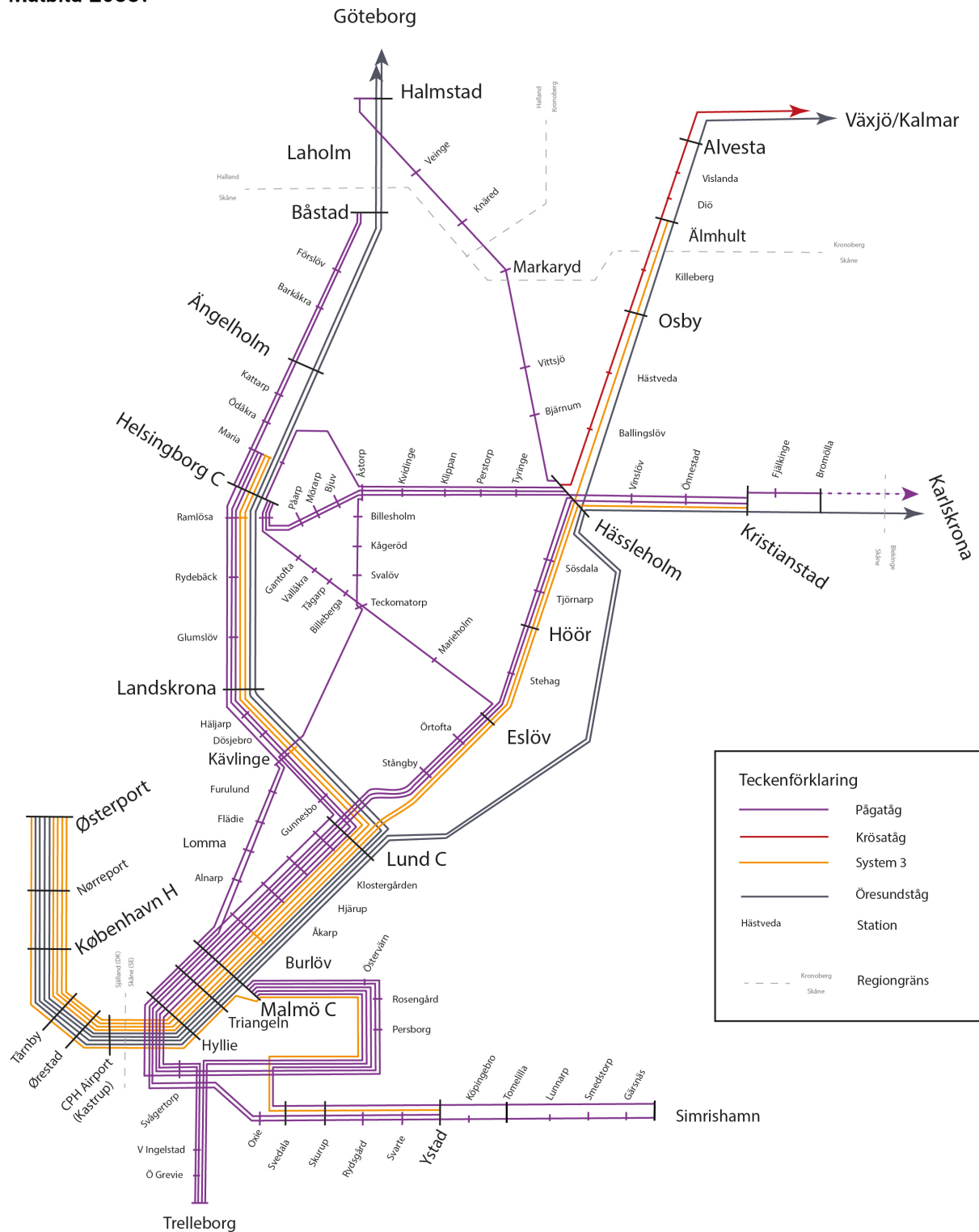
Figur 18: Schematisk bild över behov av tågtrafik för att nå målen år 2035. Exklusive fjärrtåg och godståg. En linje innebär ett tåg per timme i vardera riktningen i högtrafik.
