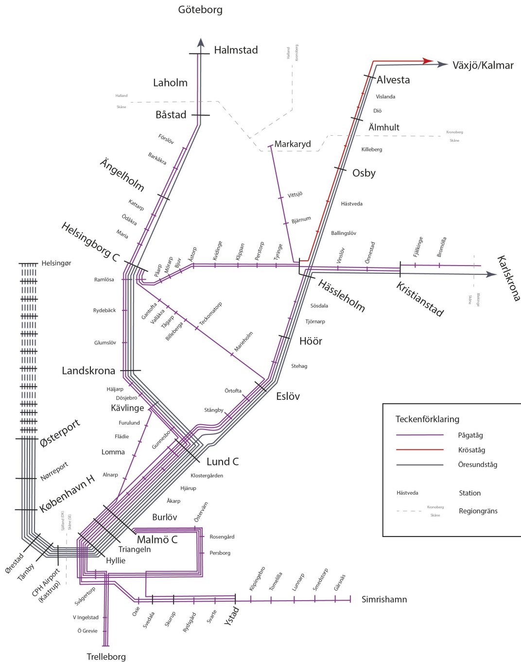
Figur 1: Schematisk bild över dagens tågtrafik (december 2020 i Skåne, exklusive fjärrtåg). En linje innebär ett tåg per timme i vardera riktningen i högttrafik.
